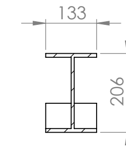
SEÇÃO F-F ESCALA 1 : 10
