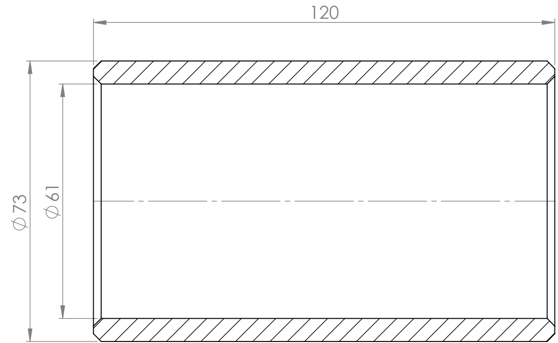
SEÇÃO G-G ESCALA 1 : 1
