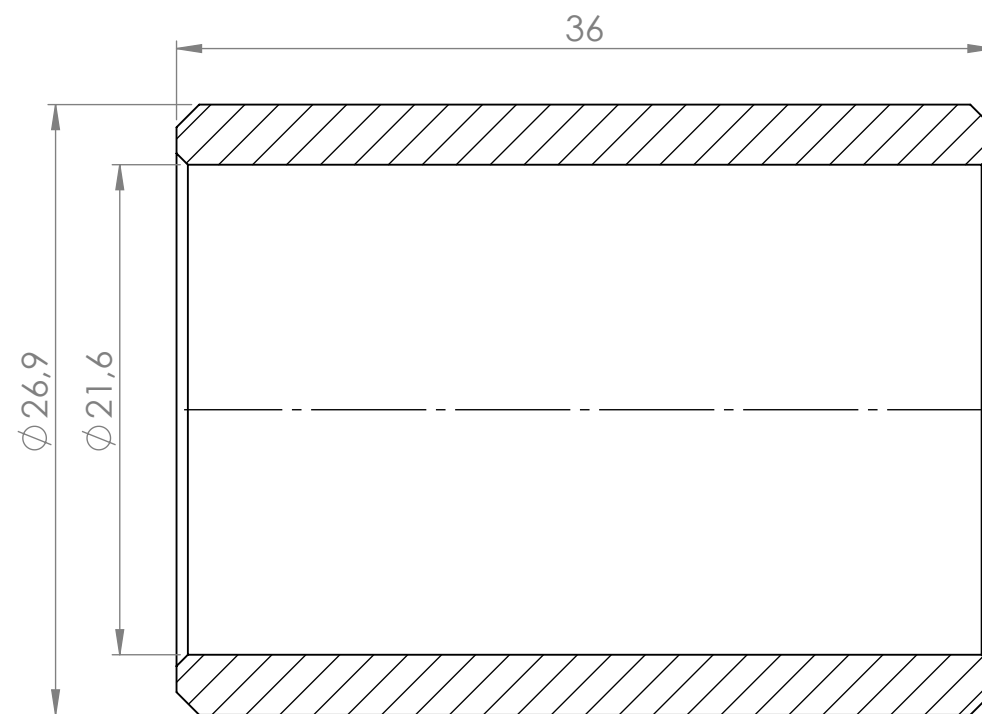
SEÇÃO Q-Q ESCALA 3 : 1
