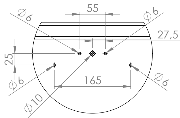
DETALHE D ESCALA 1 : 5
