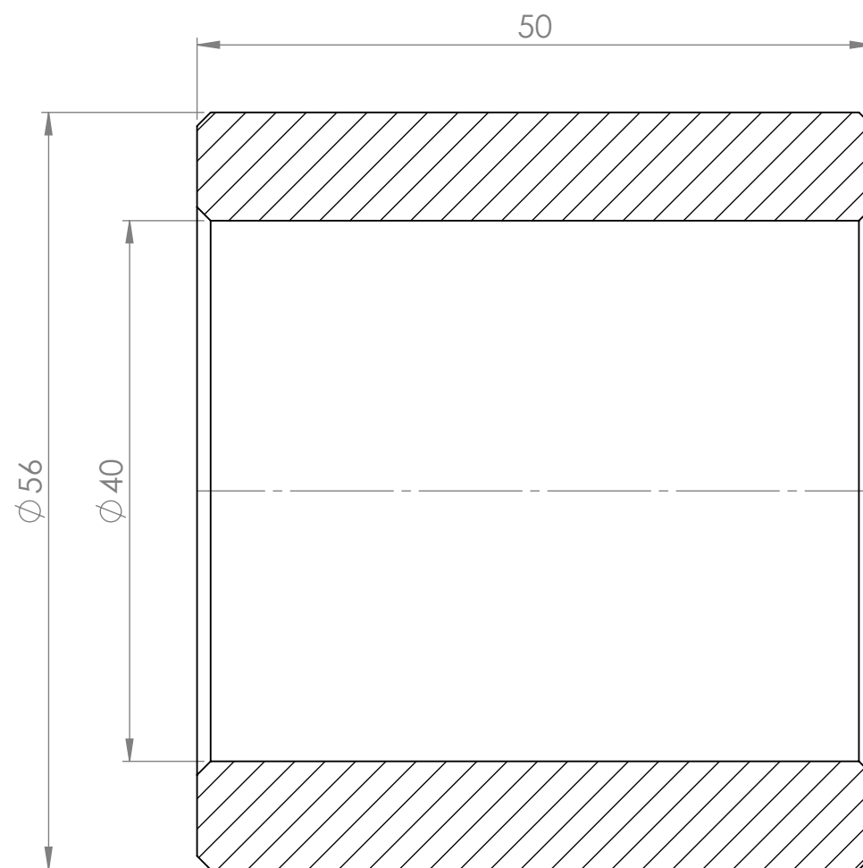
SEÇÃO G-G ESCALA 2 : 1
