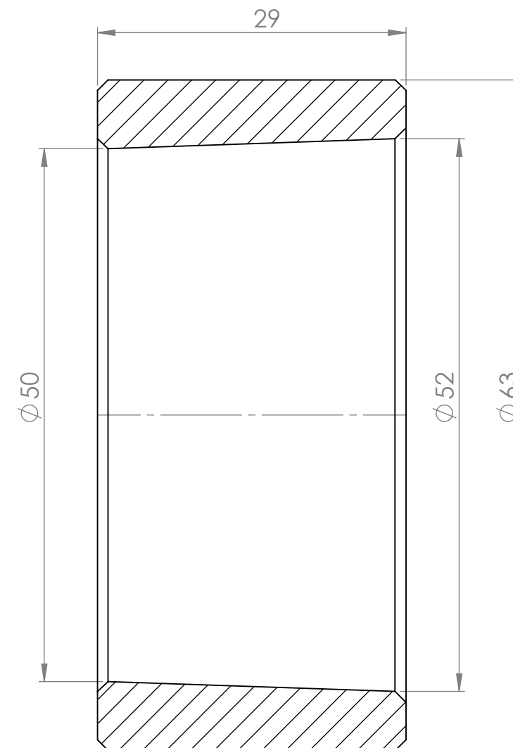
SEÇÃO H-H ESCALA 2 : 1
