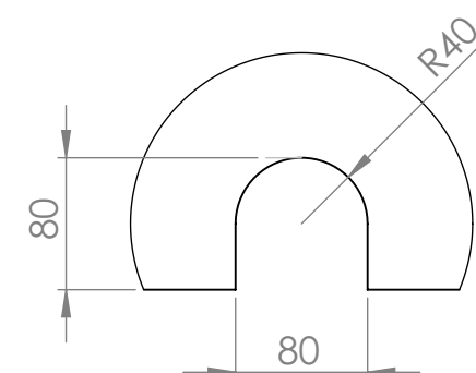
DETALHE F ESCALA 1 : 5
