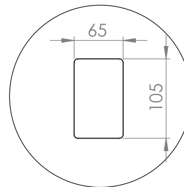
DETALHE I ESCALA 1 : 5
