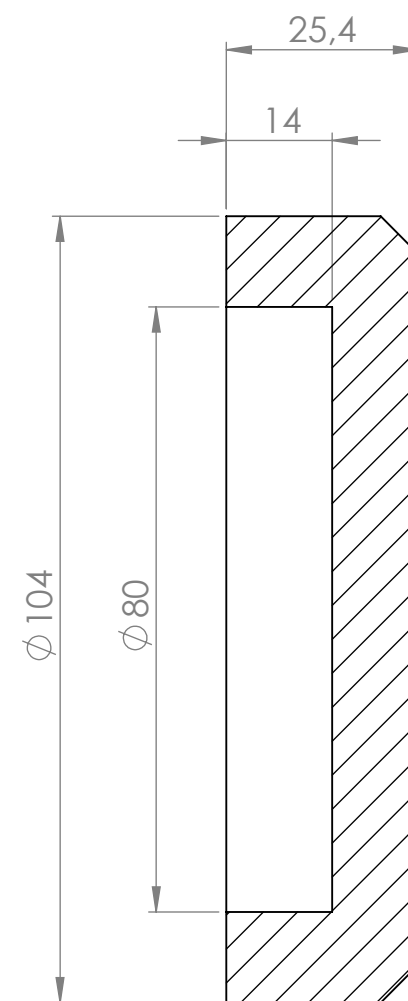
SEÇÃO A-A
