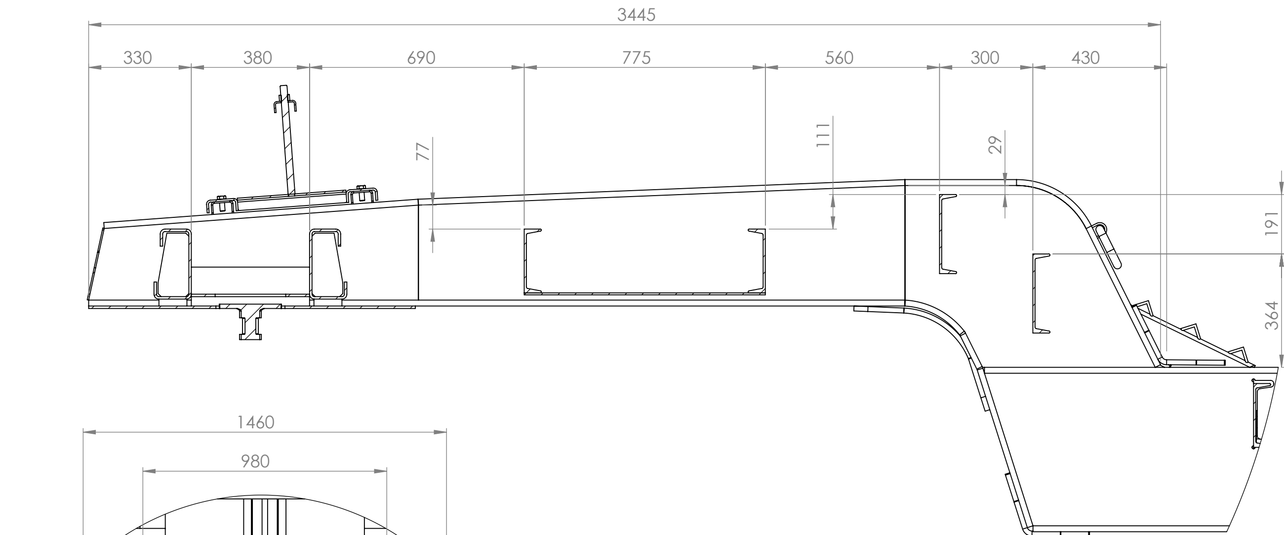
DETALHE J ESCALA 1 : 12
