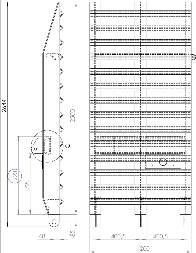
PERFIL "U" LAMINADO 8"
